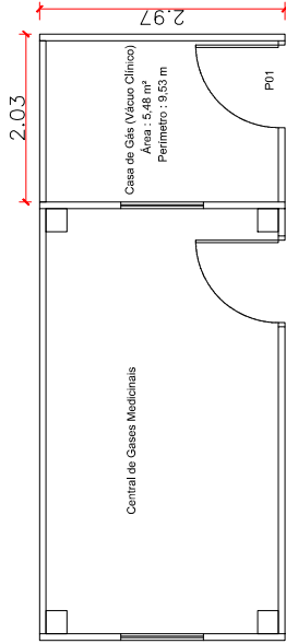
02 PLANTA BAIXA ESC.: 1/50
