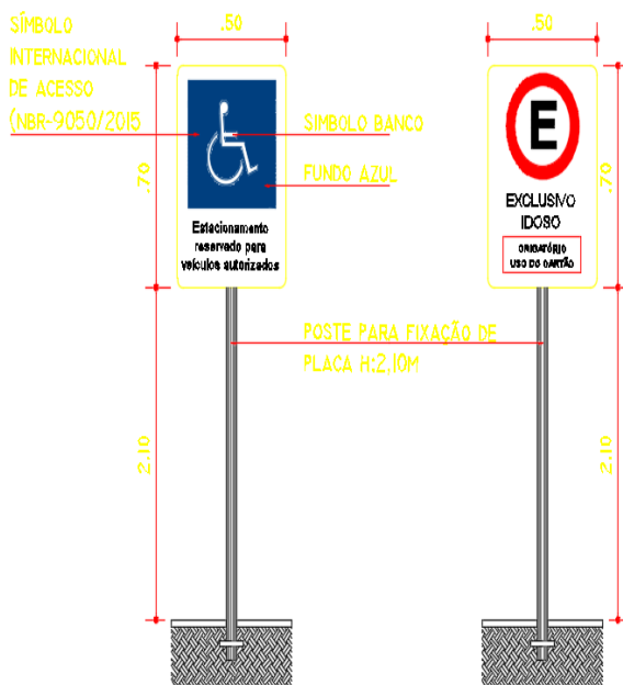
Figura 1: Detalhe de Placa Vertical de Local Acessível
