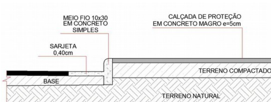
Figura 1: Meio fio em concreto pré-moldado
