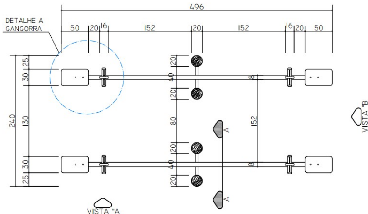
Figura 12: Gangorra
