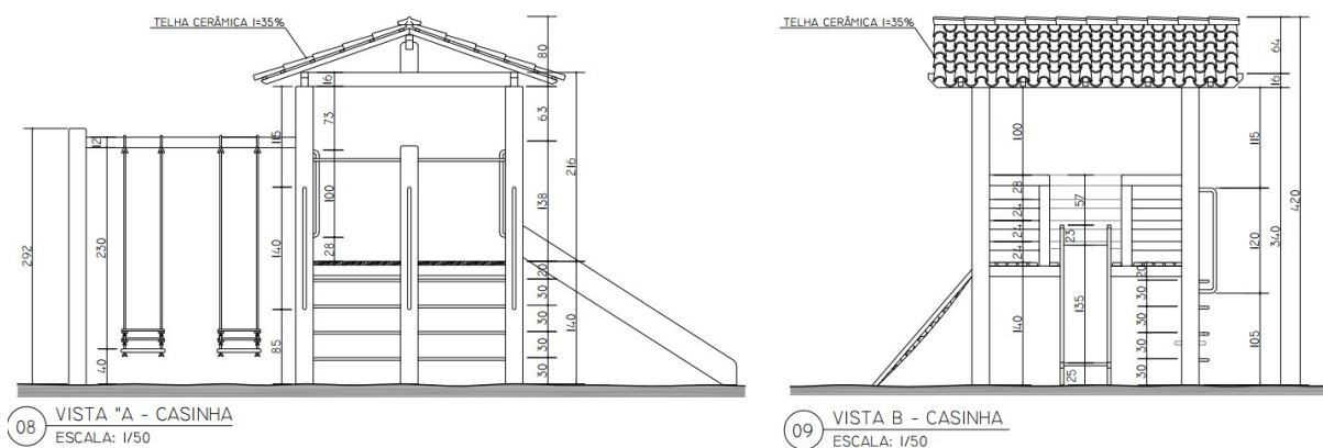
Figura 13: Casinha Multibrinquedo
